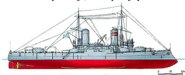
Bitevní loď «Andrej Prvozvanny» (stavba začala v roce 1905): kompletní podřízení tvaru trupu lodi taranové taktice. Stal se prototypem prvních variant tvarového řešení trupu dreadnoughtů typu «Sevastopol».
