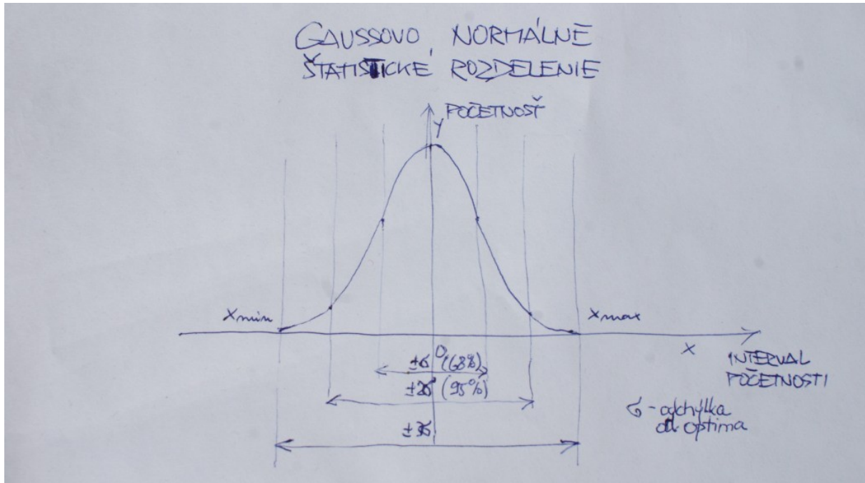
Obrazok: Gaussova krivka Normálneho štatistického rozdelenia
